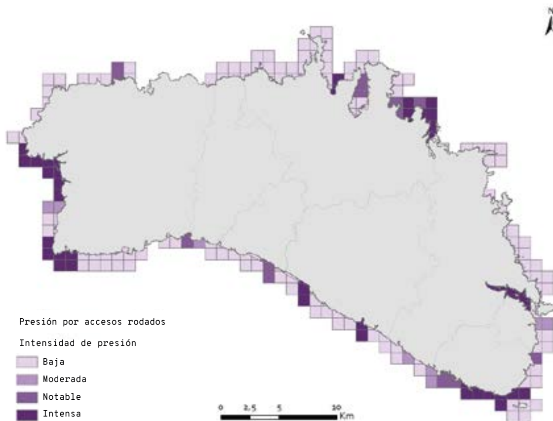
Figura 10. Mapa de Menorca representando la estima de la presión ejercida por viales rodados en el litoral. FUENTE: Bagur et al. 10
